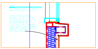
DETAIL SCALE: 1/2" = 1'-0"
